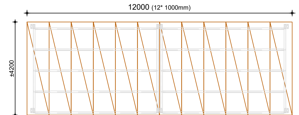
LEGPLAN VLOERPLATEN 12 stuks Vloerplaat 5.250x1.000x38 mm
