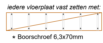
LEGPLAN VLOERPLATEN 12 stuks Vloerplaat 5.250x1.000x38 mm
