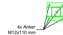
Kolom, geschoord
