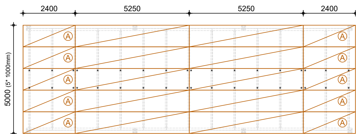
LEGPLAN VLOERPLATEN 15 stuks Vloerplaat 5.250x1.000x38 mm
