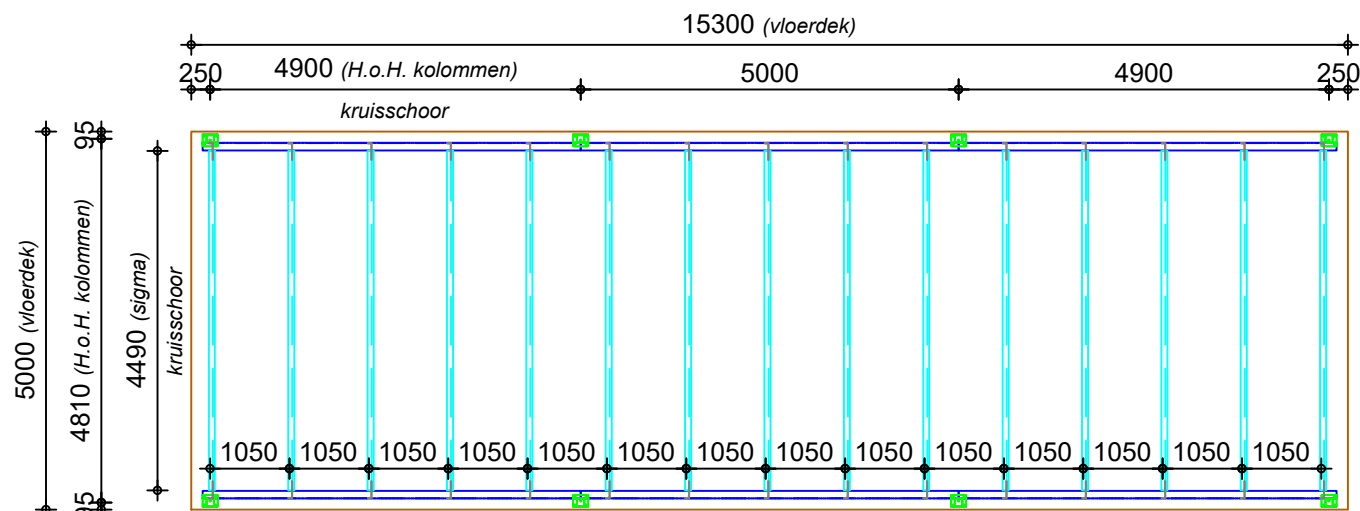
BOVENAANZICHT
