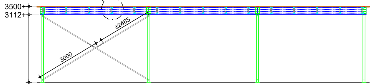
VOORAANZICHT
