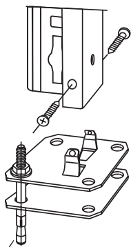
Vloeranker / Bolzenanker / Tie bolt Ancre par boulon
