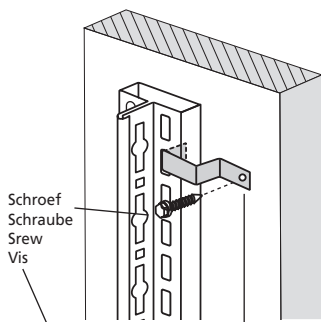
Muurbevestiging / Wandbefestigung Wall mounting / Fixation murale
