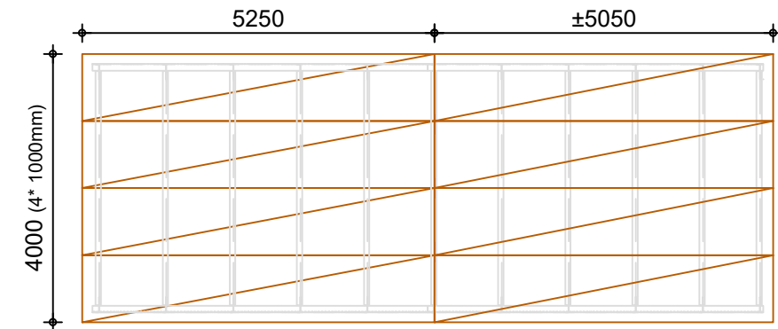
LEGPLAN VLOERPLATEN 8 stuks Vloerplaat 5.250x1.000x38 mm
